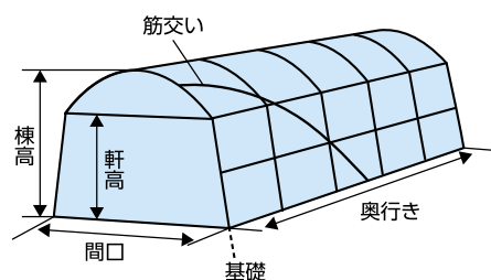
図① ハウスの構造
